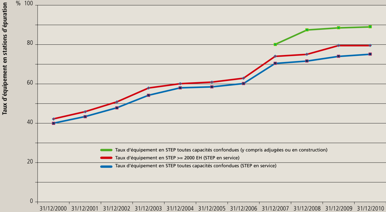
Evolution du taux d’équipement en stations d’épuration (2000 - 2010)
